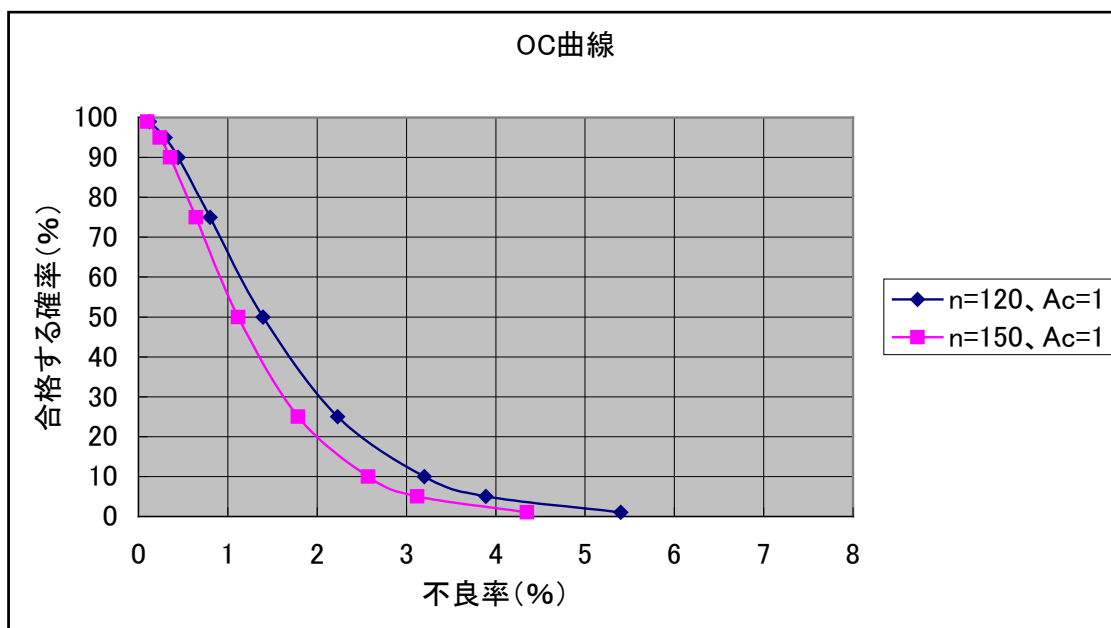
図 5-1 OC曲線
